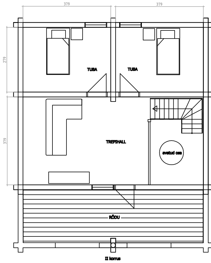
II korrus
