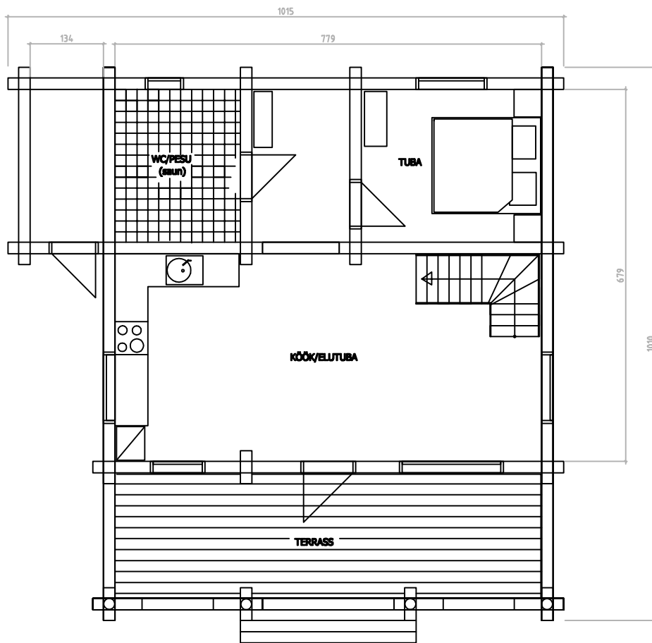
I korrus
